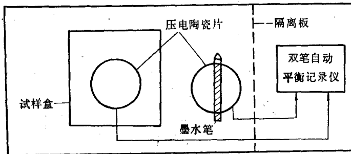
图6 压电陶瓷片试验装置示意图
